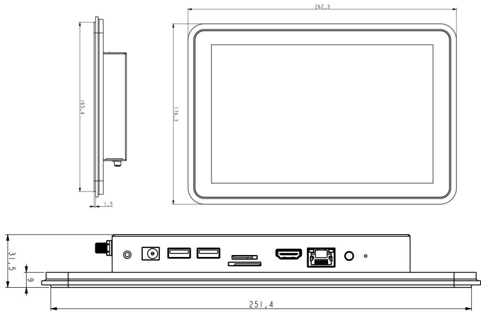
尺寸图 Dimensions (mm)
