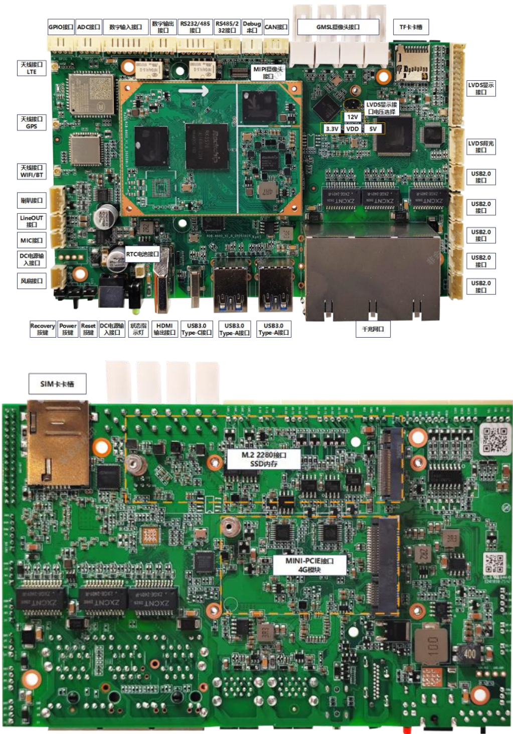
接口示意图 Interface View
