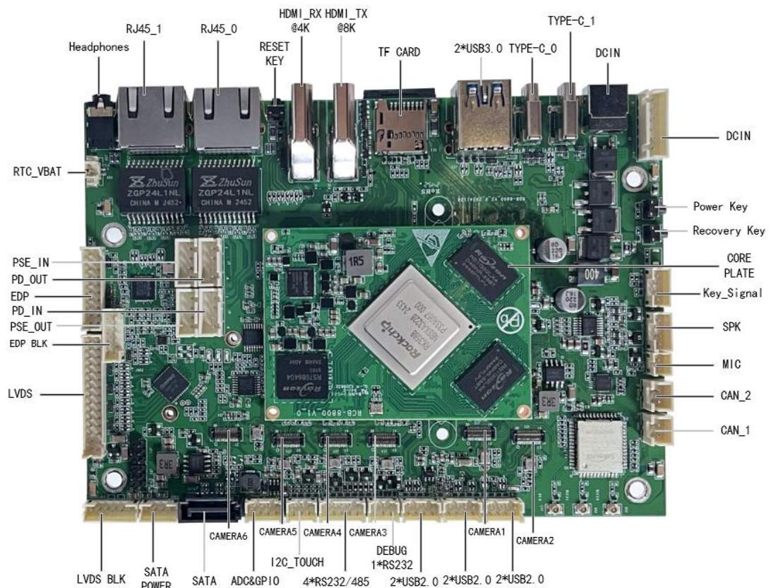
接口示意图 Interface View
