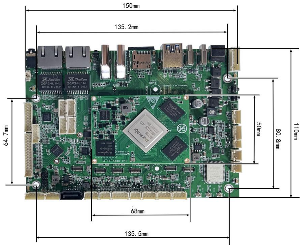
尺寸图 Dimensions (mm)
